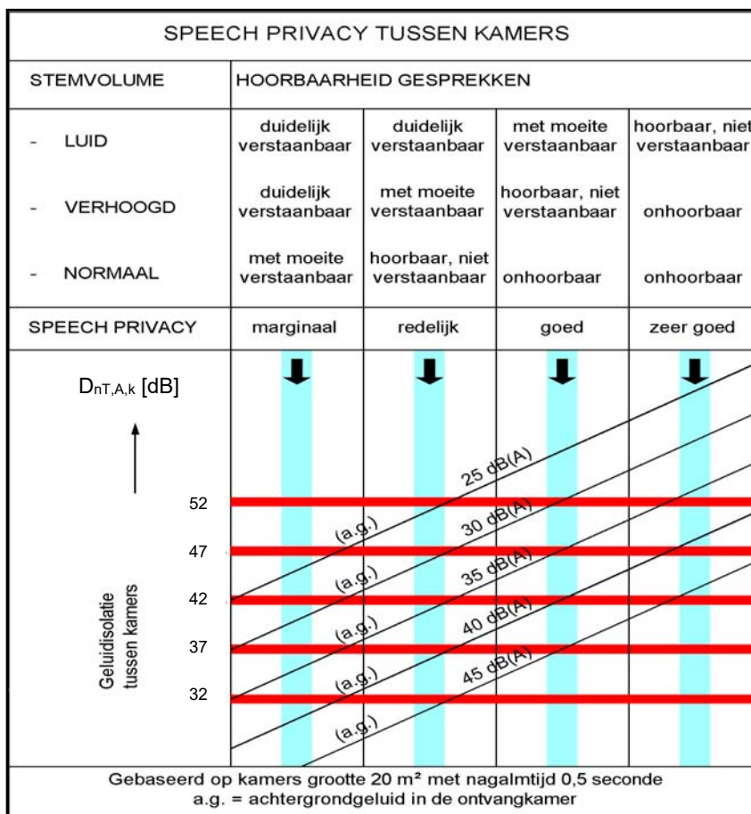
Figuur 10. Speechprivacy tussen verschillende ruimten. Af te lezen is bijvoorbeeld dat bij een geluidsisolatie van 52 dB en een achtergrondgeluidniveau in de ontvangstruimte van 30 dB(A) een goede speechprivacy is bereikt. (Let op: In plaats van D_{nT,A} wordt hier de geluidsisolatie uitgedrukt in D_{nT,A,k} .)
