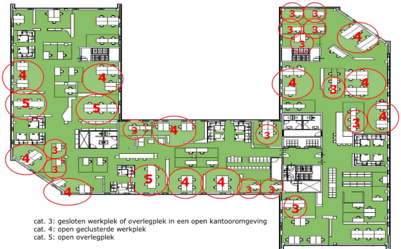
Figuur 11. Voorbeeld van akoestische prestatieniveaus categorieën 3 t/m 5.
